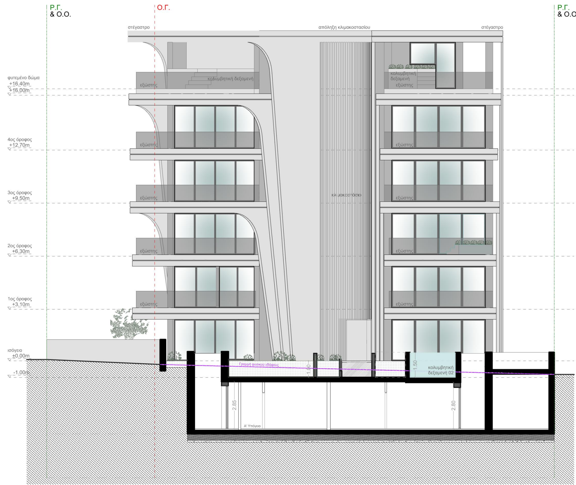
ΠΡΟΣΟΨΗ Α - Ε
